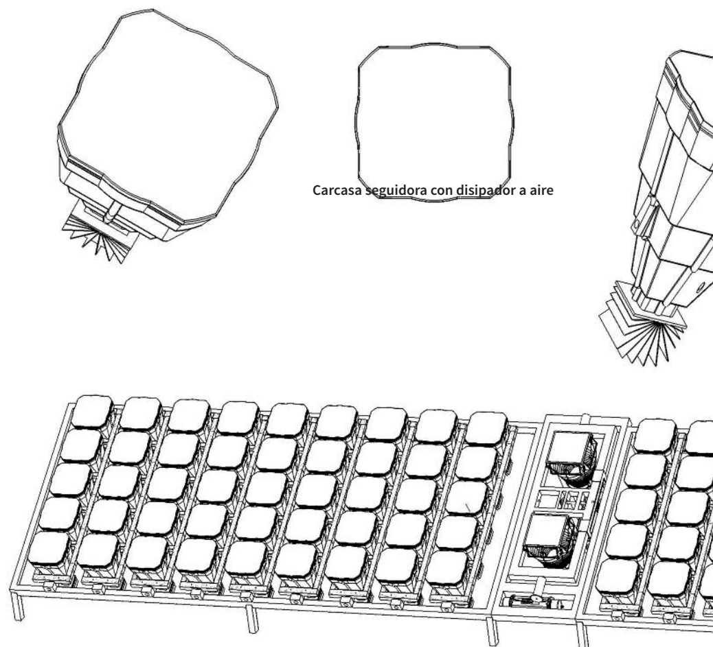
Vista 3D del módulo SOLARAYS definitivo formado por 9x5x2 seguidoras, Pmáx (W eléctricos)= 992 W , Pmáx (W térmicos)=1.444 W
